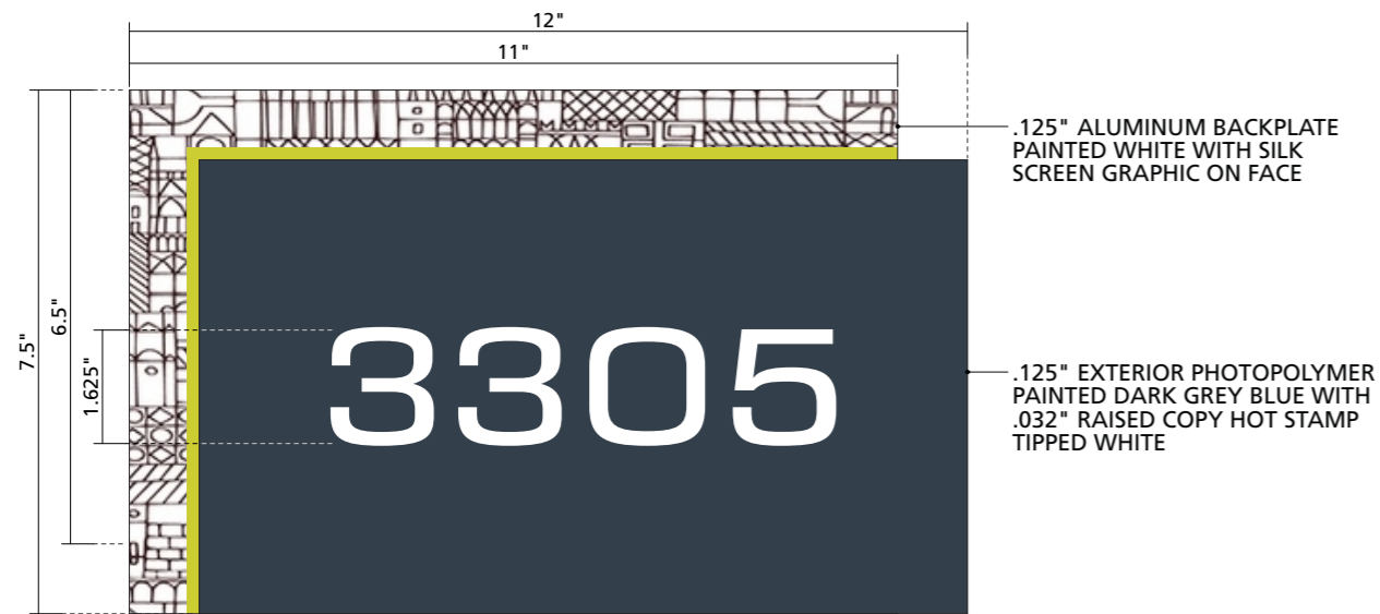
EXTERIOR BUNGALOW ID scale: 4" = 1'-0"
