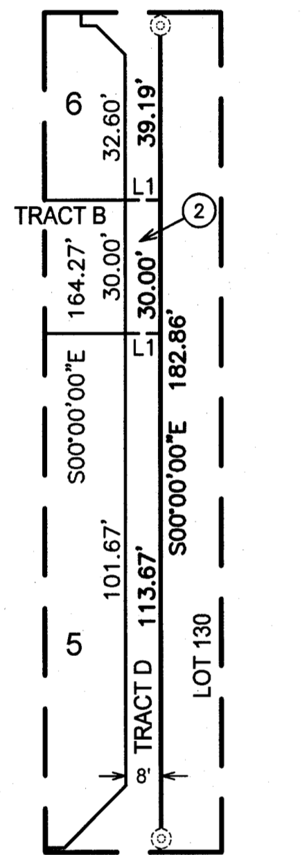
DETAIL 'C' (SCALE: 1" = 30')
