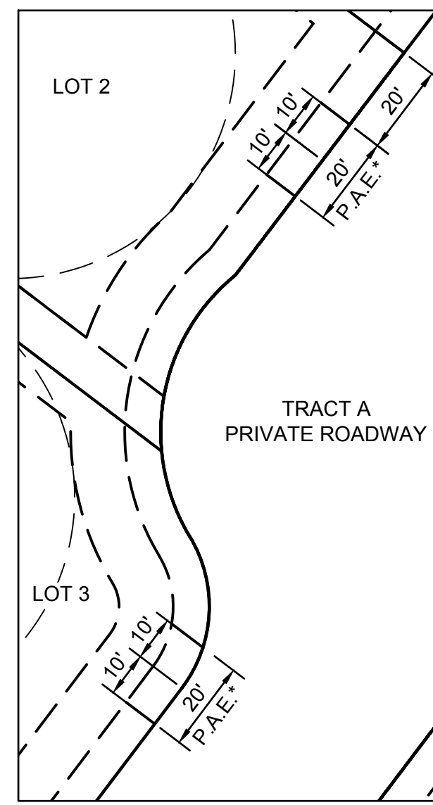
DETAIL "B" SCALE: 1" = 30'
