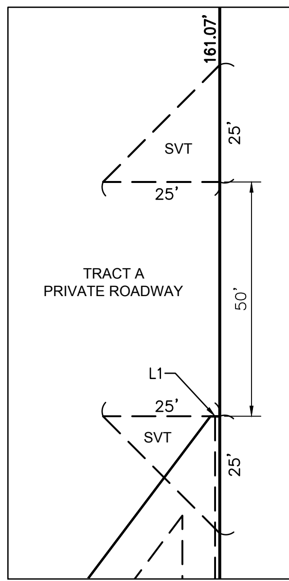
DETAIL "A" SCALE: 1" = 20'
